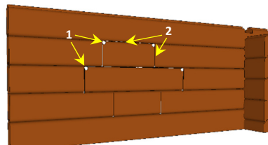
2. Skær de udvalgte bjælker væk, (bor huller (1) og skær (2) med en stiksav) med forskydning ind i den friske del af bjælkerne. (De kan fjernes flere end anvist på tegningen). Pas på vindpap, vand- og el-installationer!
