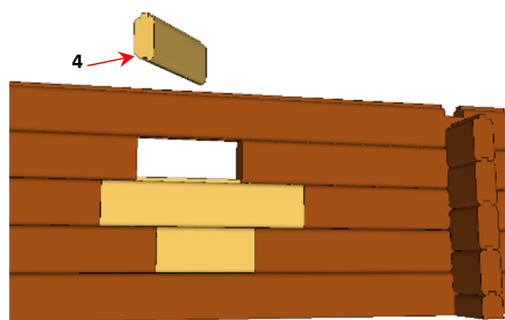
4. I øverste bjælke skal bagnet (4) skæres væk, så væggen lukkes.
