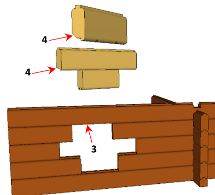
3. Fjern resterne af den gamle not (3). Herefter lukkes huller med de nye bjælker som anvist.
