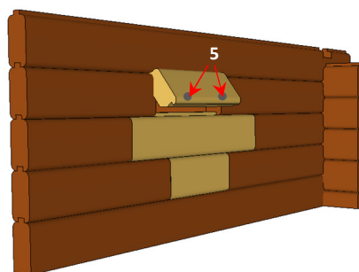
5. Til sidst skubbes øverste bjælke på plads og skrues (5) den fast.
